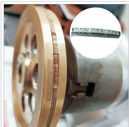
Die Embossing
